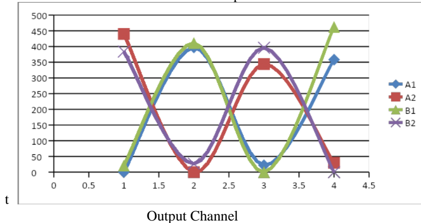
Gambar 5. Grafik Nilai Intensitas Cahaya Pada Tiap Output Port
